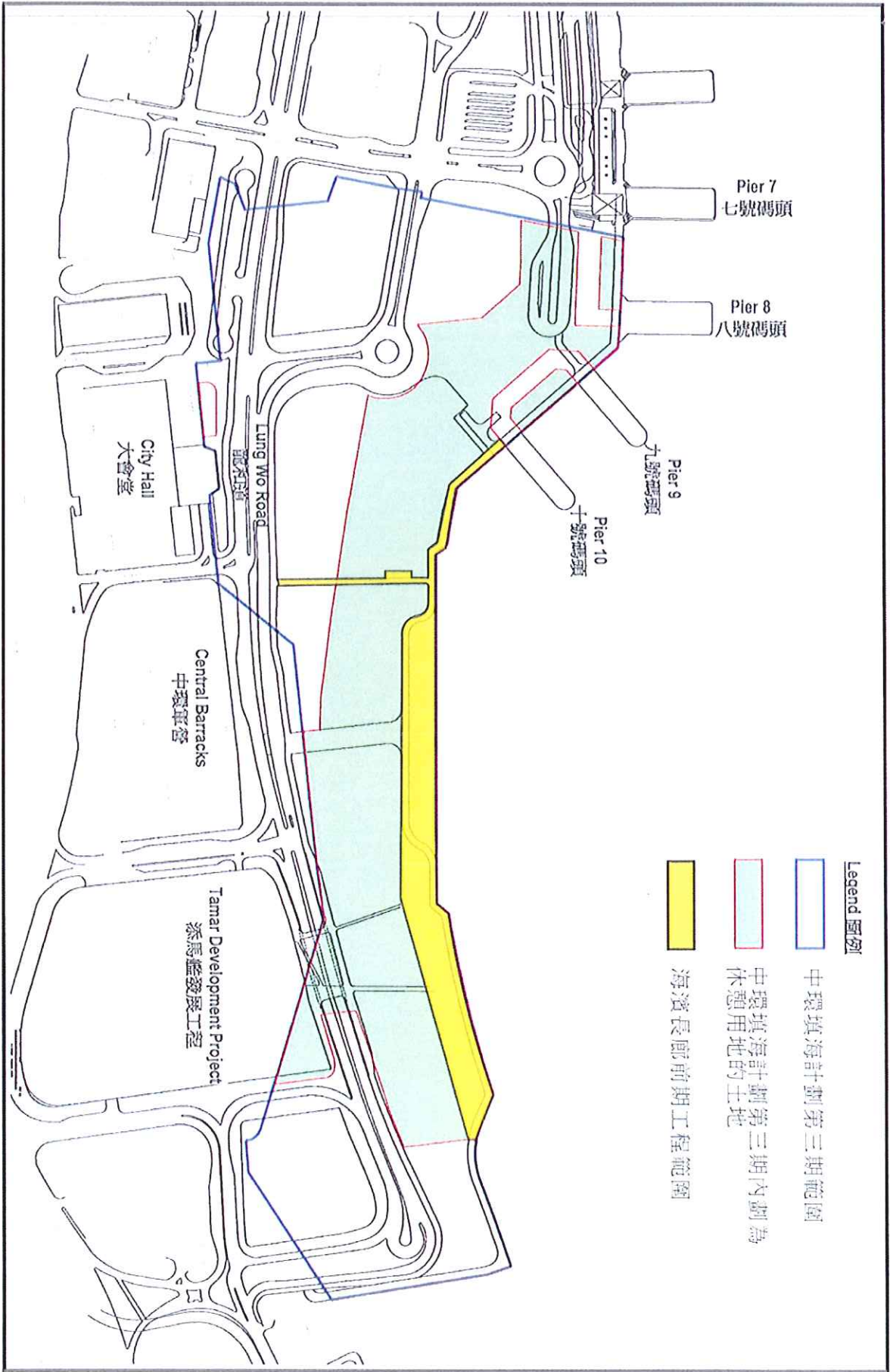
建議海濱長廊前期工程休憩用地命名為「中西區海濱長廊 - 中環段」的位置圖
