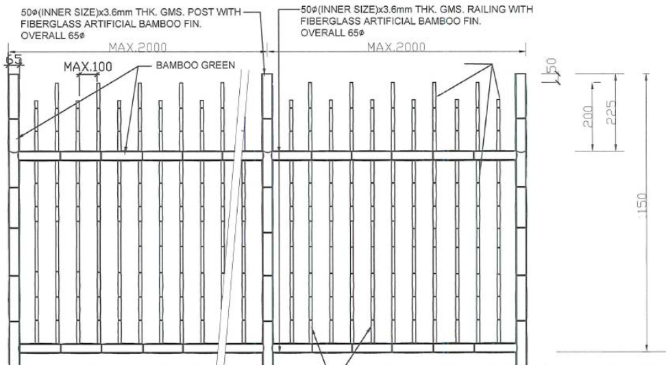
籬笆設計圖
