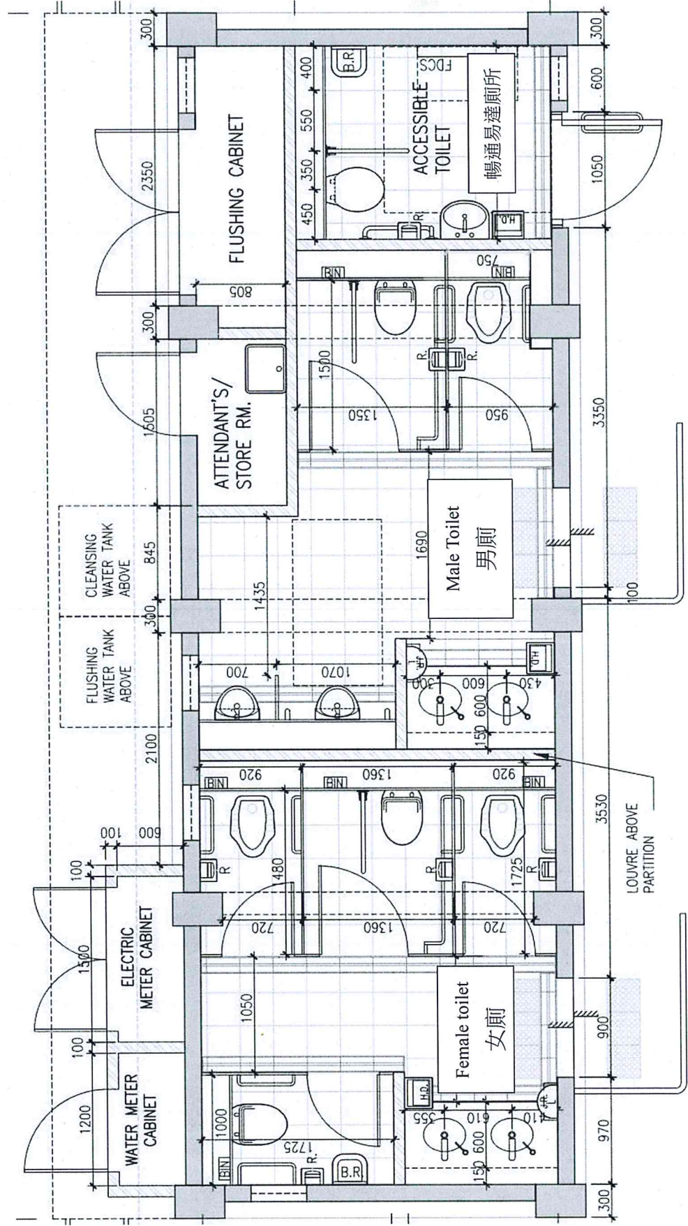
男廁、女廁及暢通易達廁所平面圖
