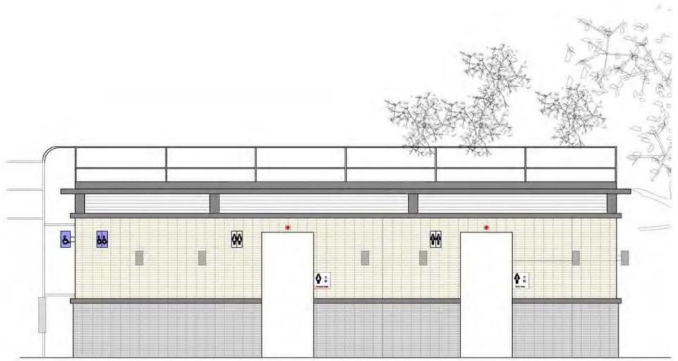
南面立面圖 (正面) SOUTH ELEVATION (FRONT)
