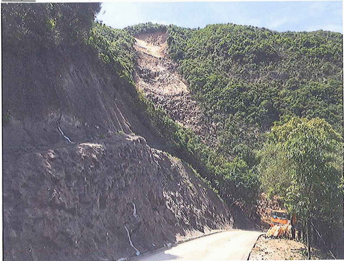
附圖四：西貢西灣路的山泥傾瀉情況（二）
