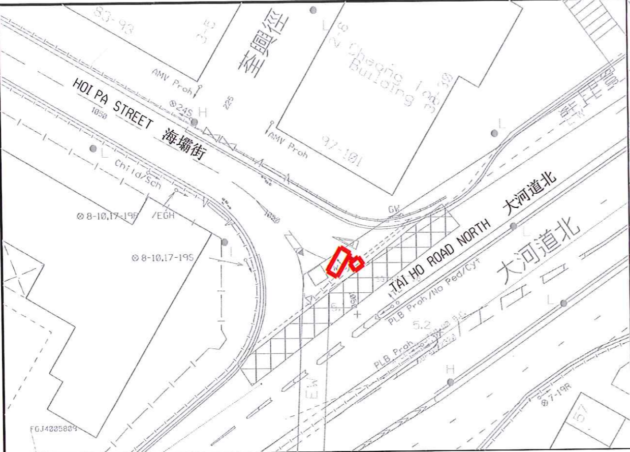
PROPOSED DWF1 AT HOI PA STREET 擬建造的旱季截流器 - 海壩街
