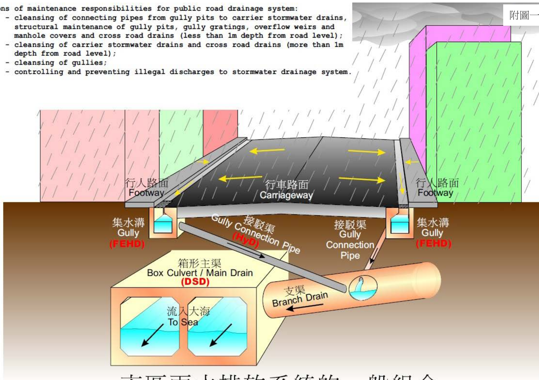
市區雨水排放系統的一般組合 Typical Layout of Urban Stormwater Drainage System
