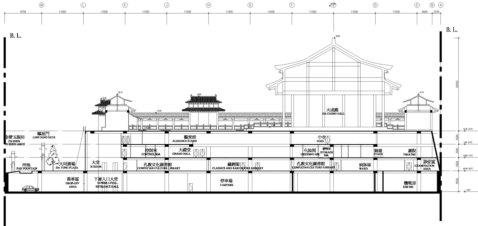
A - A 剖面圖 SECTION AA'
