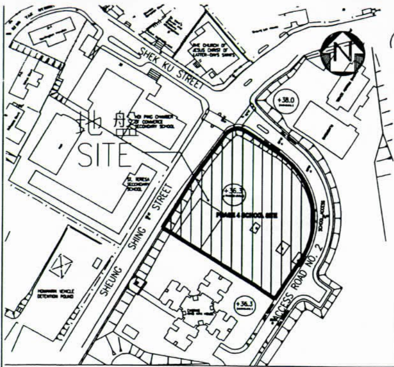
位置圖 LOCATION PLAN
