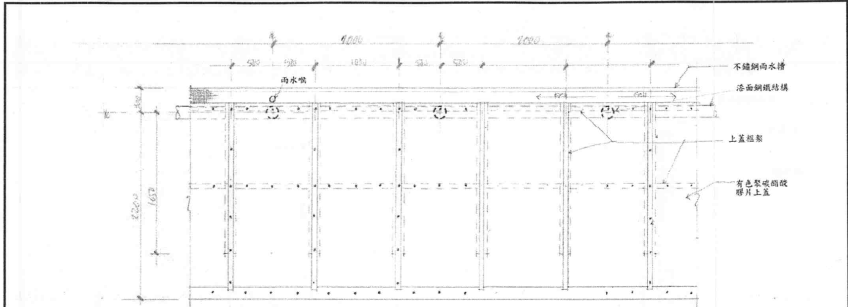
行人路上蓋(在天橋上)平面圖; 支柱間距: 2米
