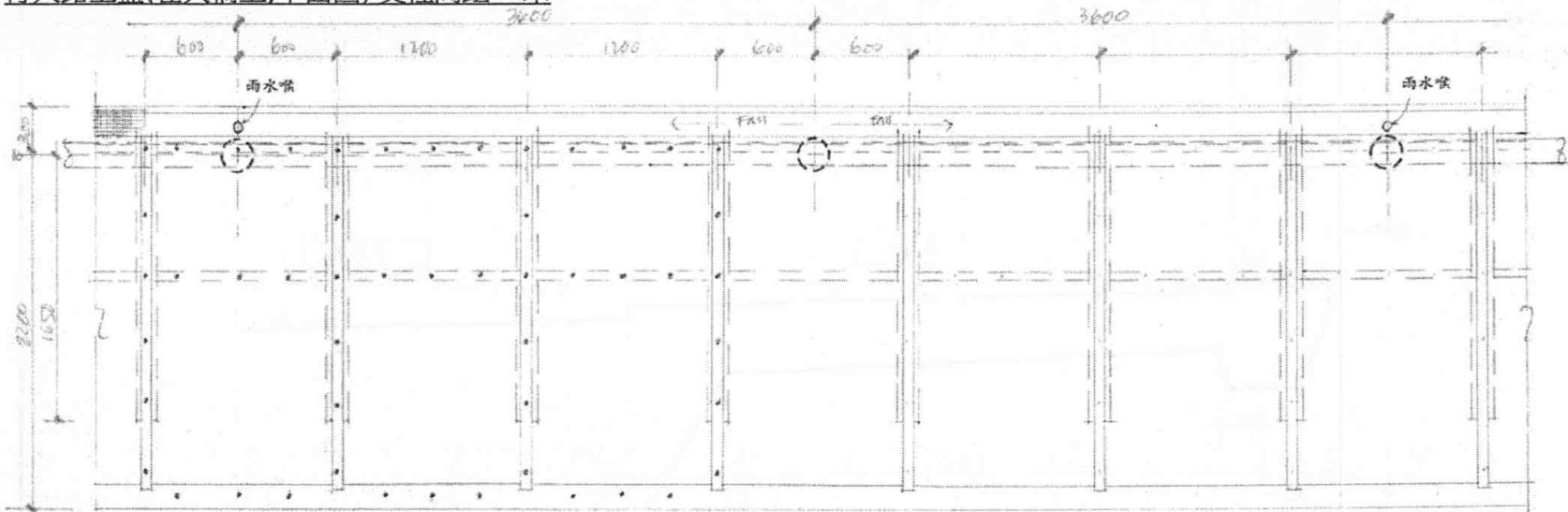
行人路上蓋(在天橋外)平面圖; 支柱間距: 3.6米
