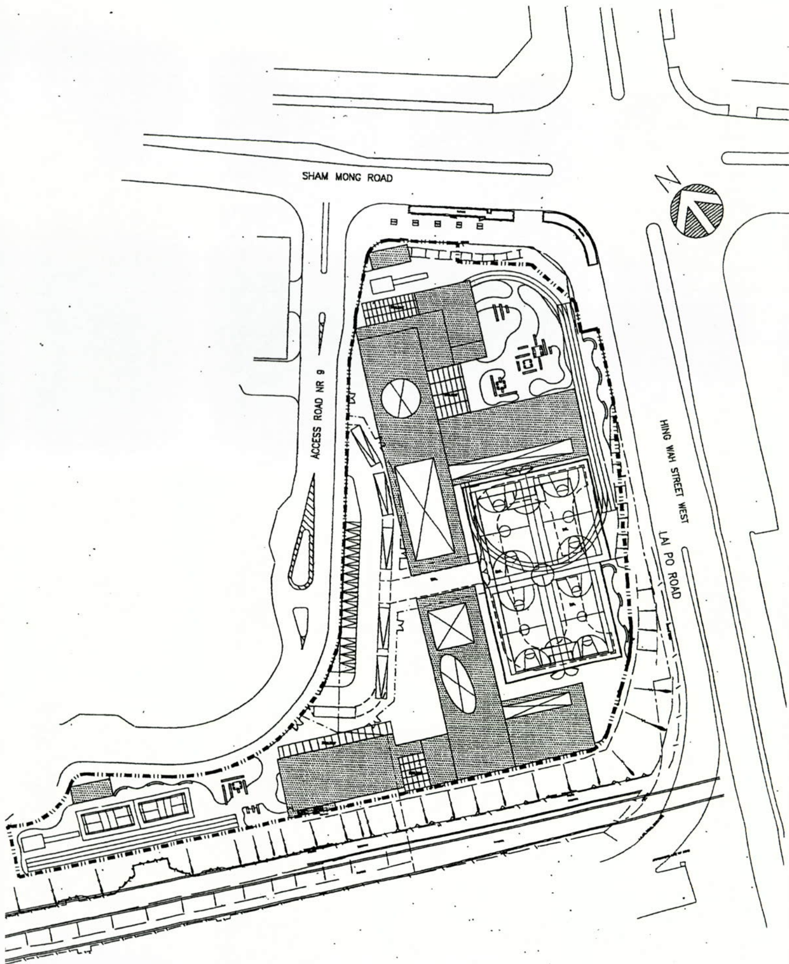
圖一：西九龍填海區第十號地盆一所小學(3319EP) 及一所中學(3256ES)的校舍設計平面圖
