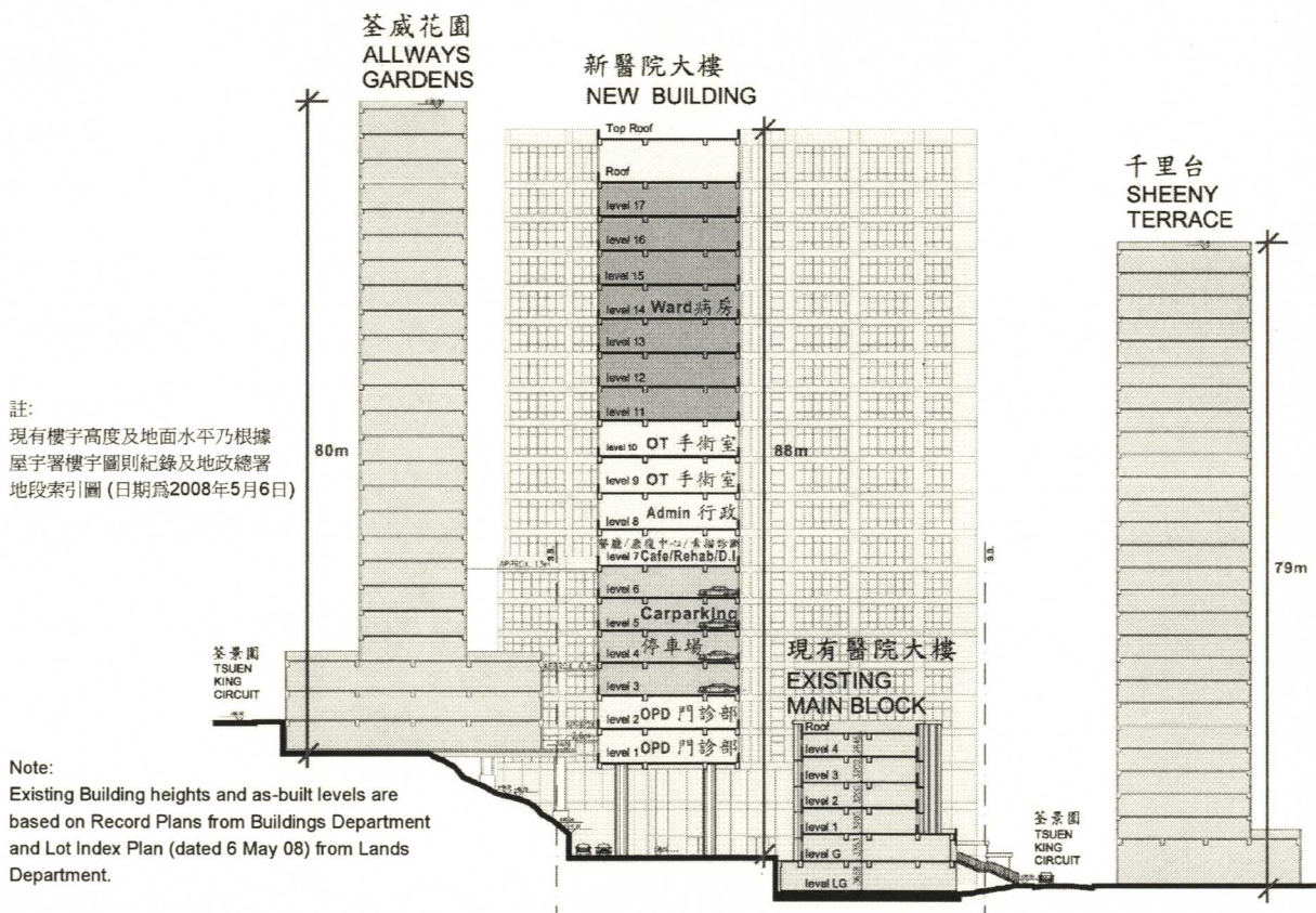
Section 剖面圖
