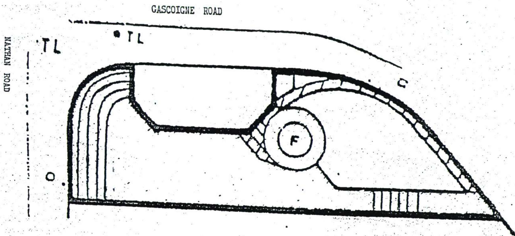
普慶廣場花園平面圖 Layout Plan of Astor Plaza Garden (面積：0.052公頃)
