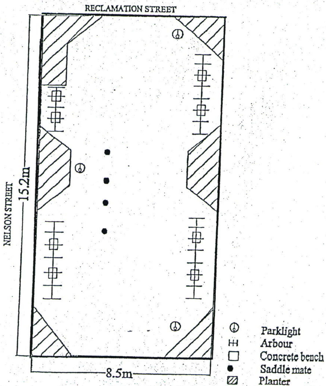
新填地街/奶路臣街休憩處平面圖 Layout Plan of Reclamation Street / Nelson Street SOA
