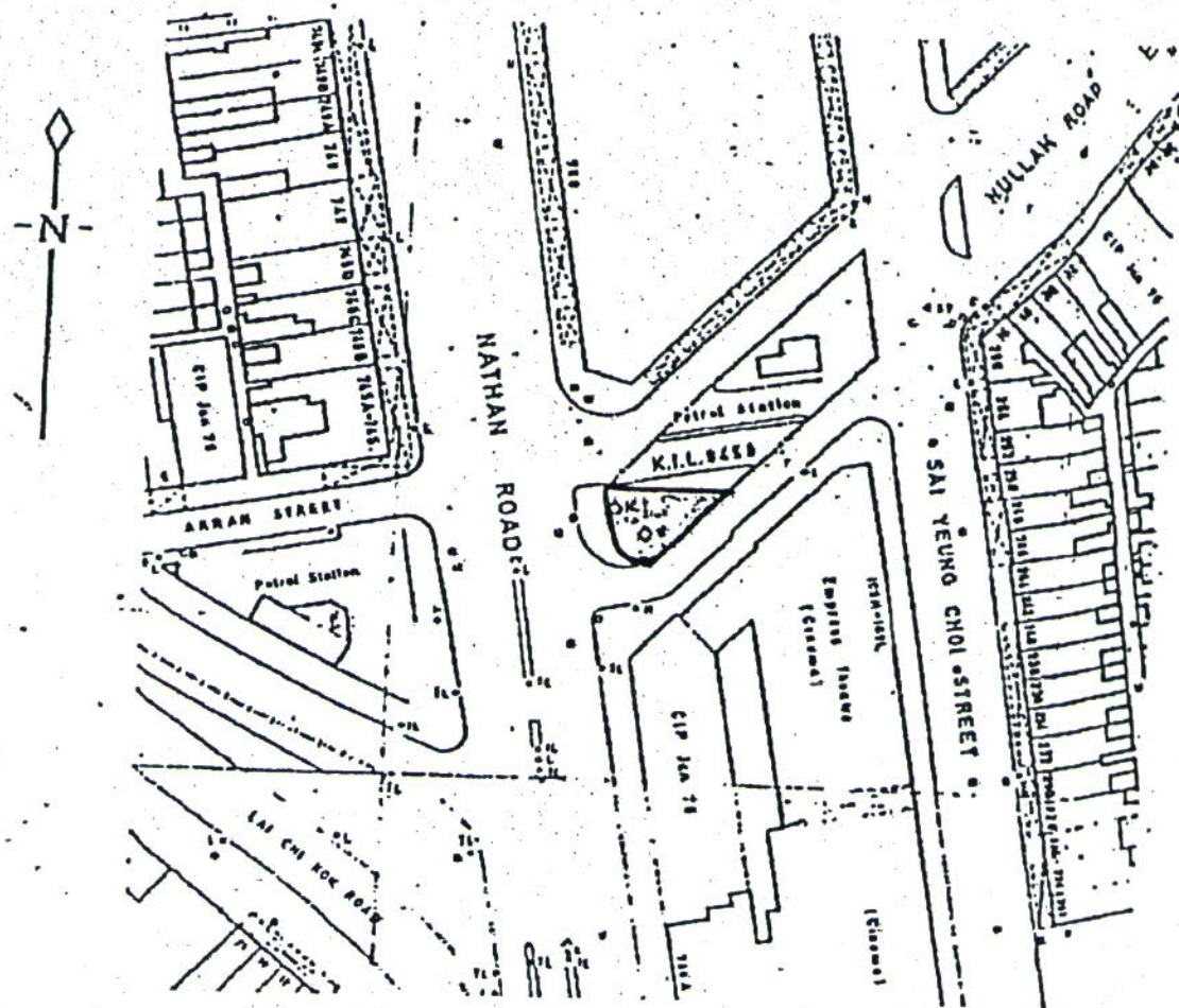
水渠道休憩處平面圖 Layout Plan of Nullah Road SOA
