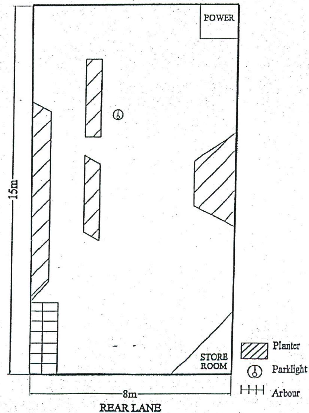
廣東道/奶路臣街休憩處平面圖 Layout Plan of Canton Road / Nelson Street SOA
