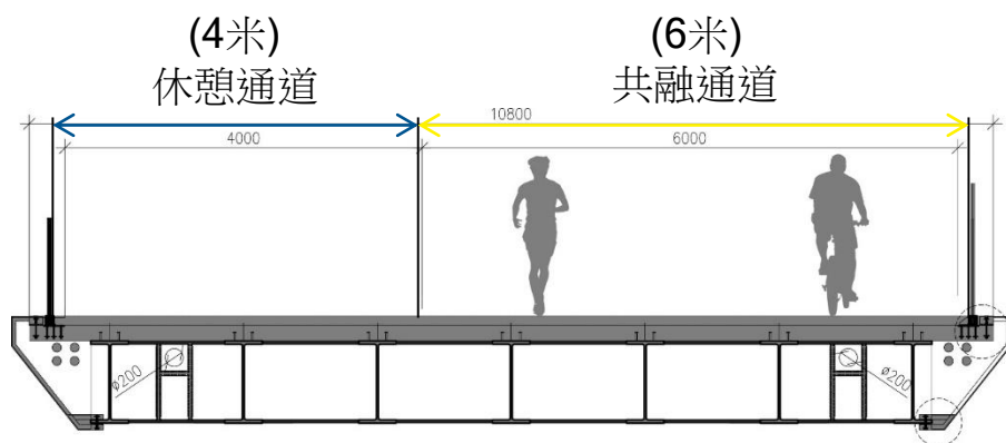
典型剖面圖
