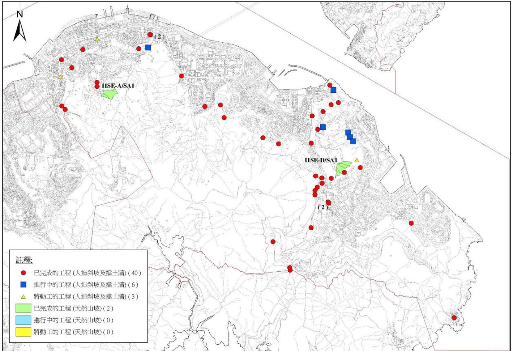
東區的長遠防治山泥傾瀉工程位置圖
