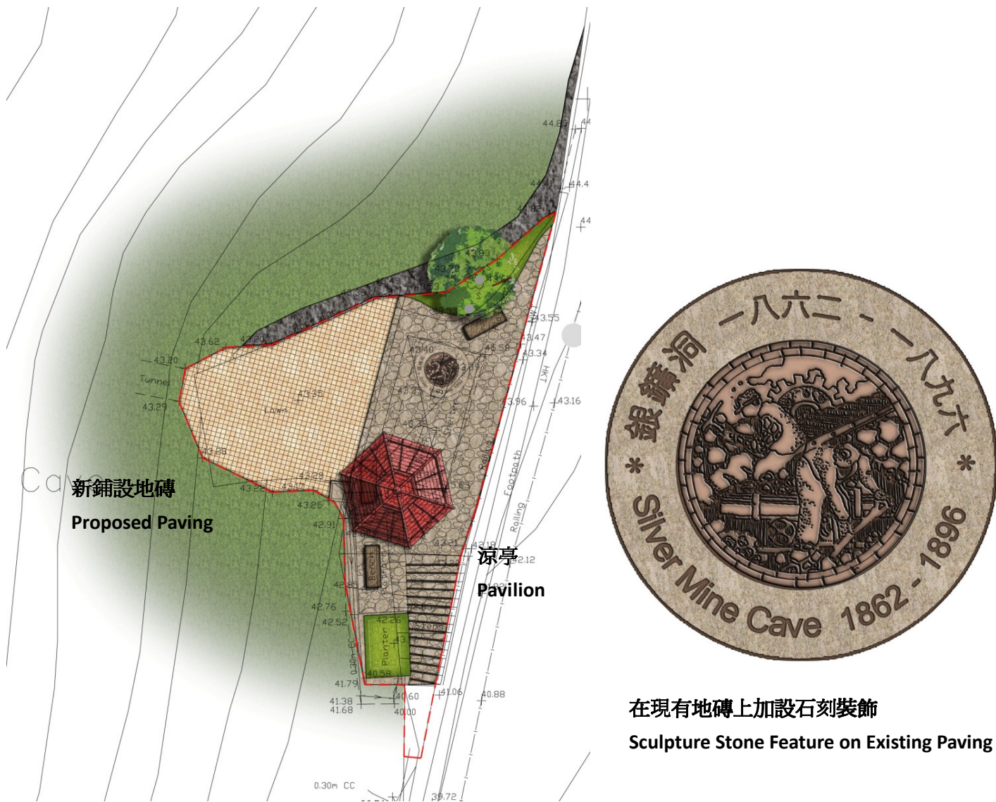
附圖三 擬建銀鑛洞休憩區的平面圖
