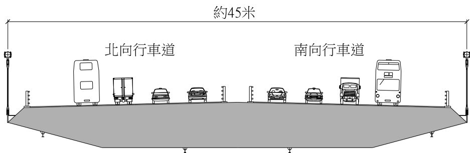
青龍大橋剖面圖
