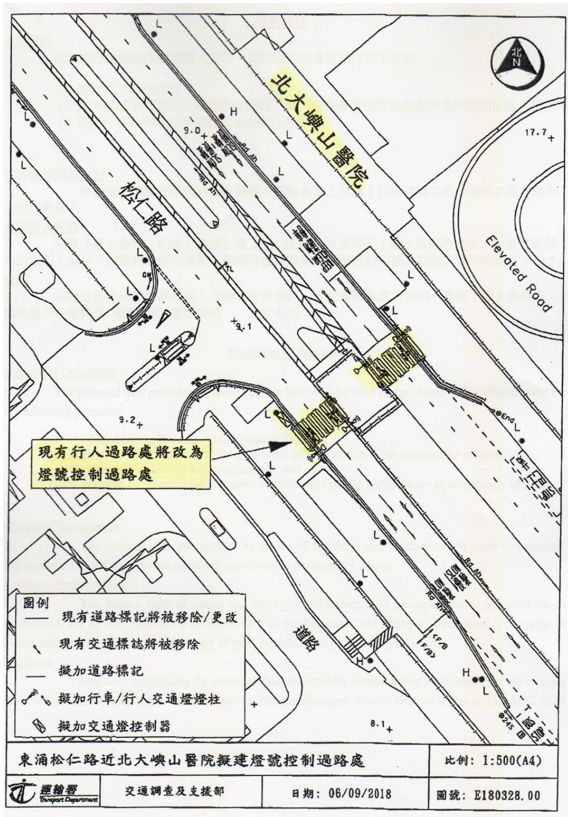
附圖四：松仁路近北大嶼山醫院位置的行人過路處增設安全交通燈的草圖
