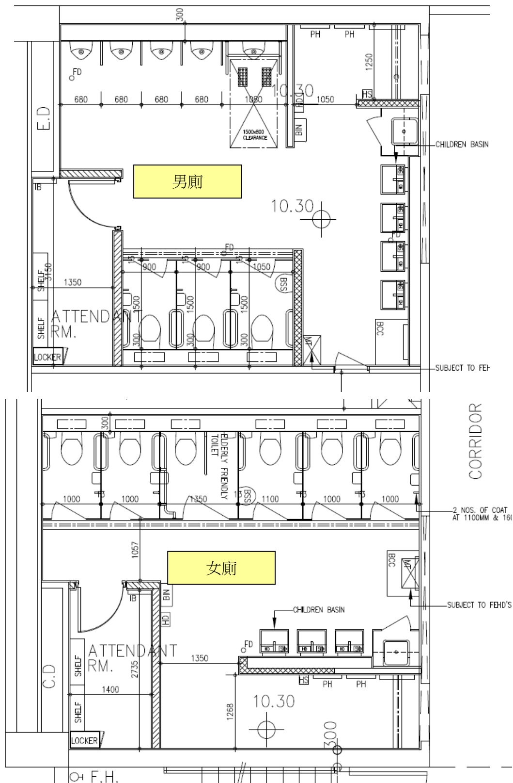
紅磡市政大廈公廁閣樓平面圖(工程後)
