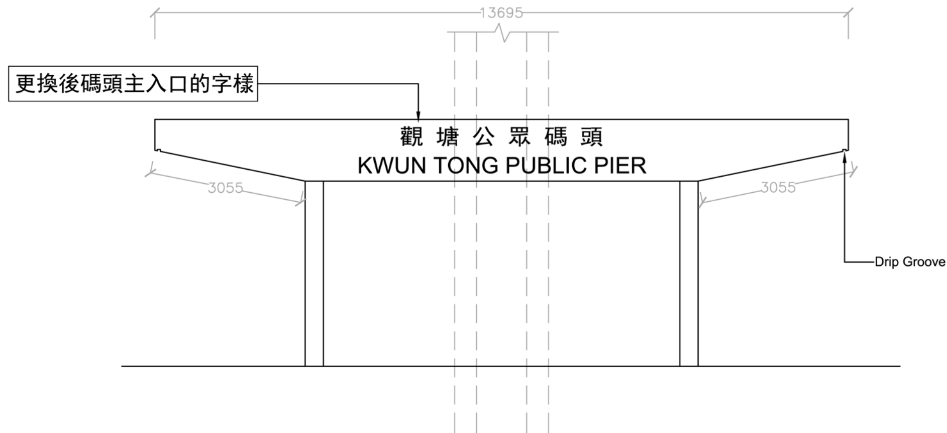
立面圖 A
