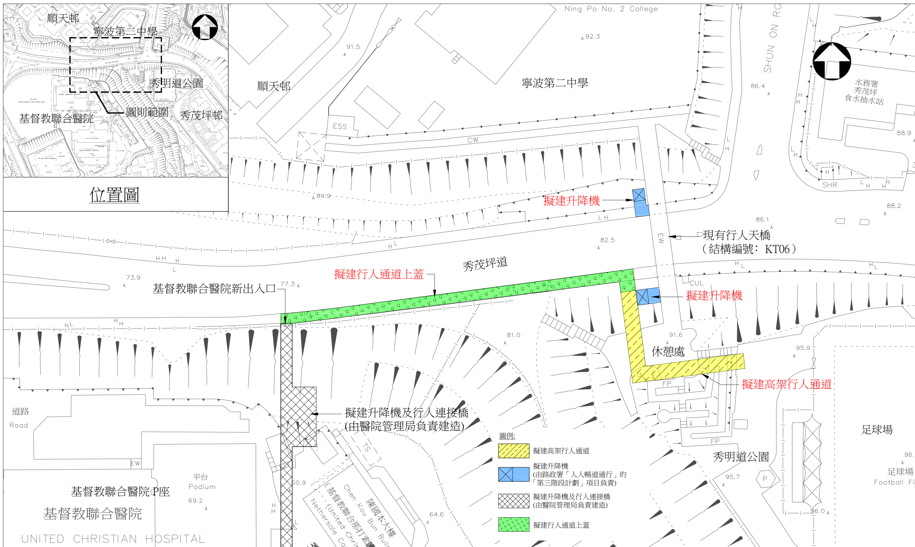
附圖 連接秀茂坪道和秀明道公園的升降機及行人通道系統 - 平面圖
