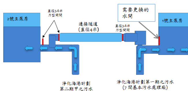
圖 C 第一階段施工程序 (2018 年 2 月)
