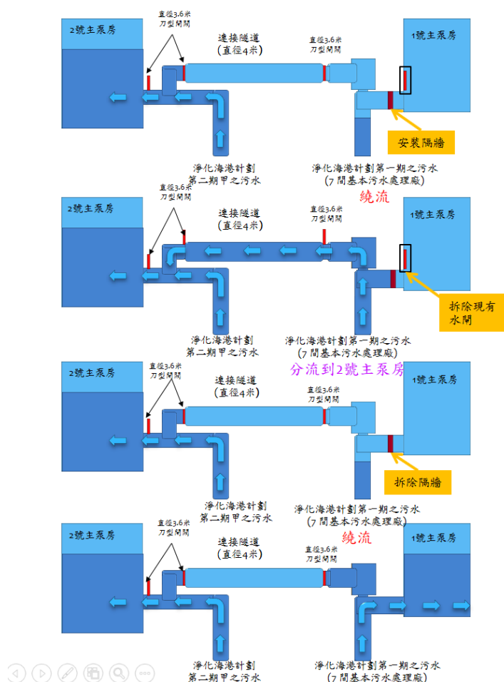
圖 D 第二階段施工程序（2018/19 年旱季）
