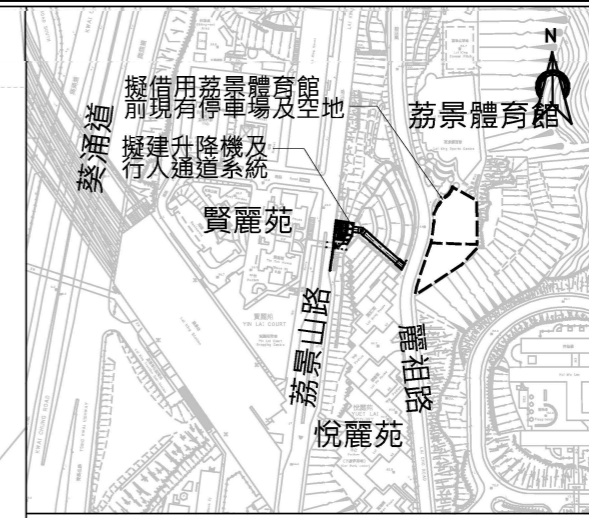
位置圖 KEY PLAN
