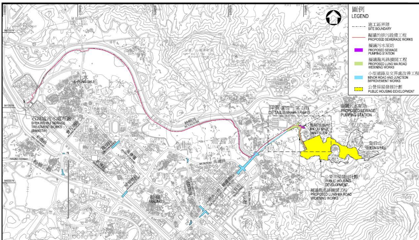
工務計劃項目編號 783CL 粉嶺皇后山發展之基礎設施工程 PWP ITEM NO. 783CL INFRASTRUCTURE WORKS FOR DEVELOPMENT AT QUEEN'S HILL, FANLING 工地平面圖 SITE PLAN 比例 SCALE 1:20 000
