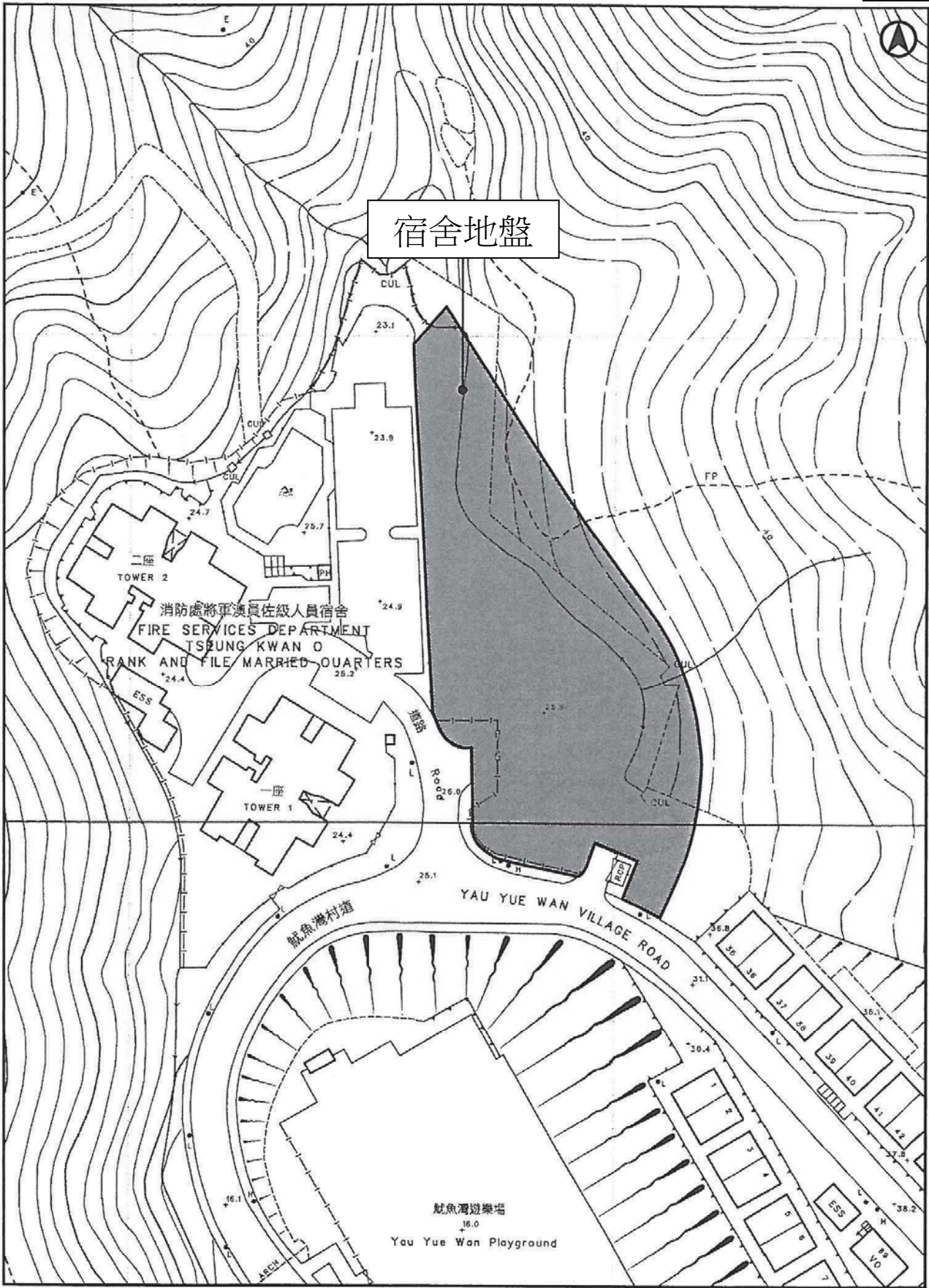
將軍澳魷魚灣村道香港海關宿舍建造工程 圖則二
