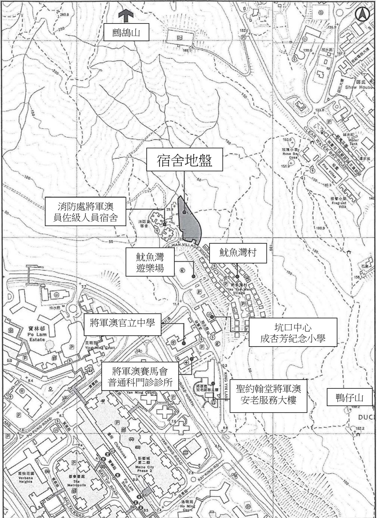
將軍澳鯨魚灣村道香港海關宿舍建造工程 圖則一
