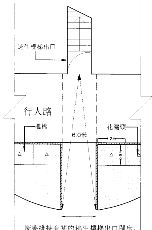
放大位置圖
