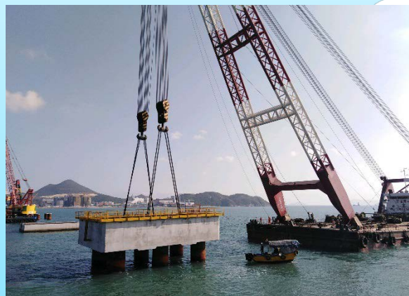
跨灣連接路主橋建造工程
