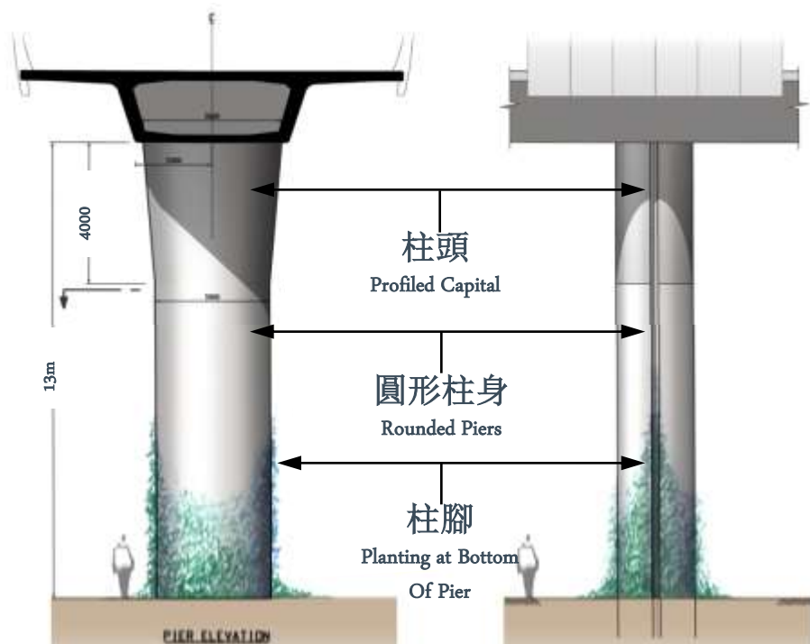
正面圖 Front Elevation
