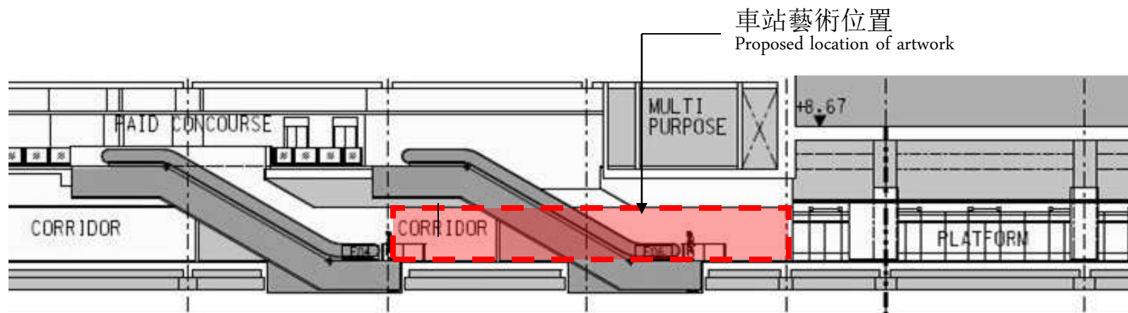
剖面圖 Section
