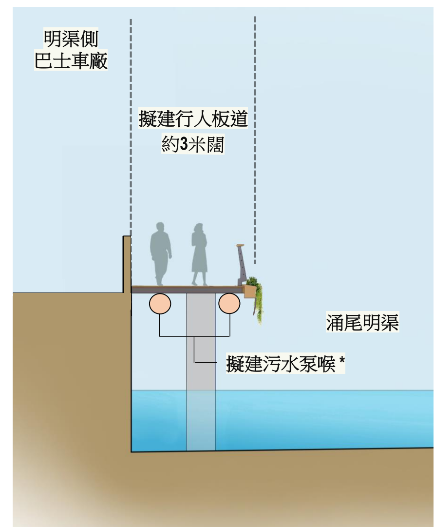
剖面甲-甲'
