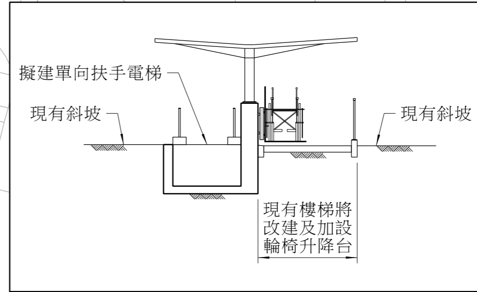
擬建單向扶手電梯系統切面參考圖 (待詳細設計完成後確定)
