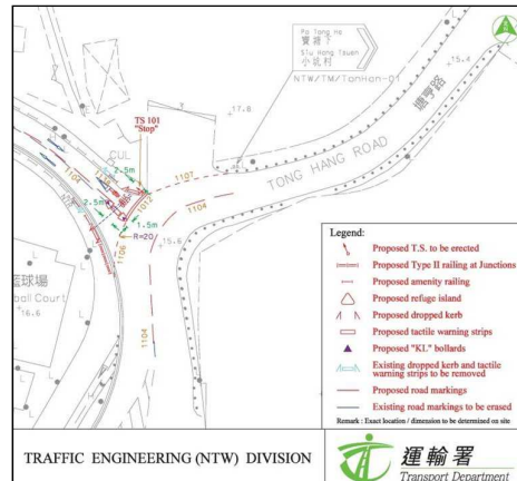
設計圖
