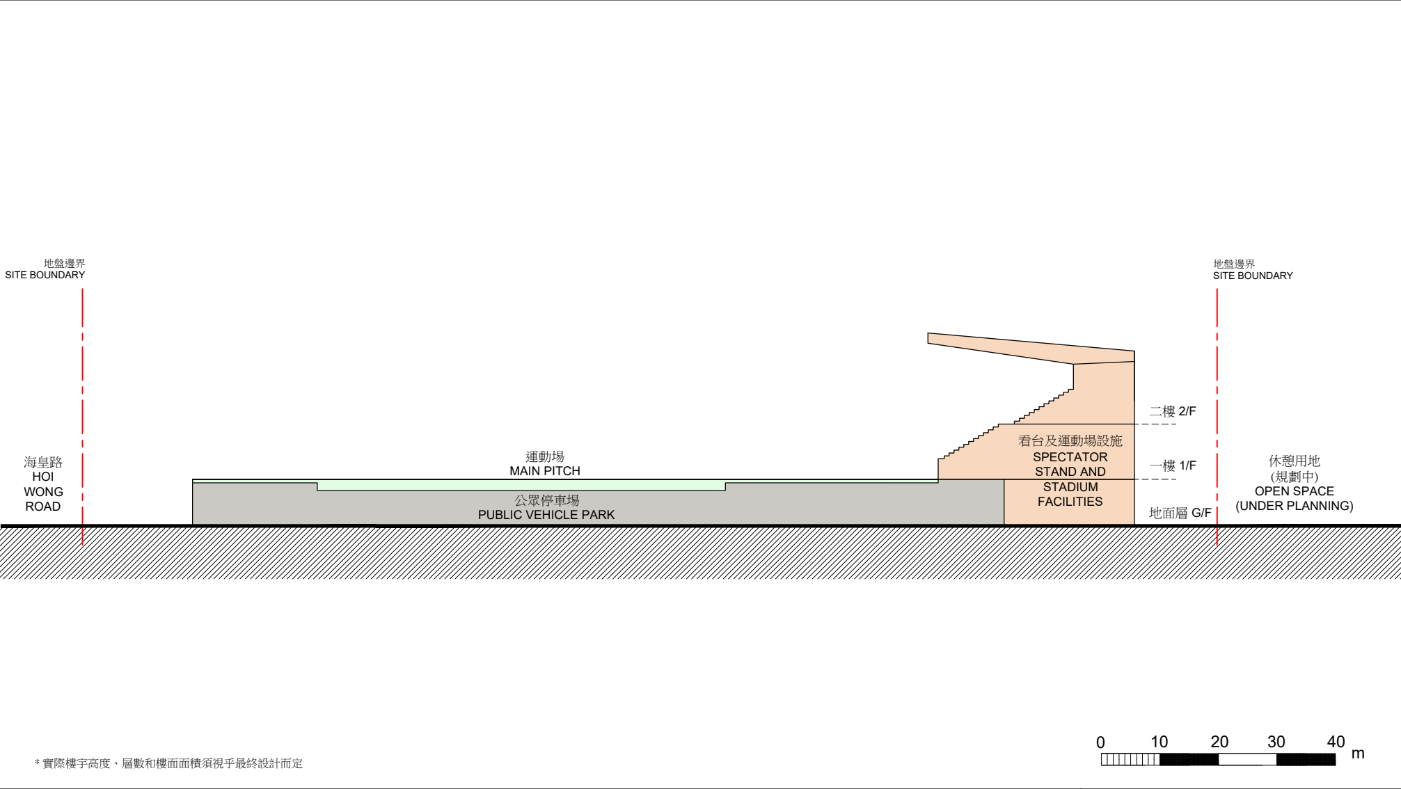
剖面圖 SECTION A
