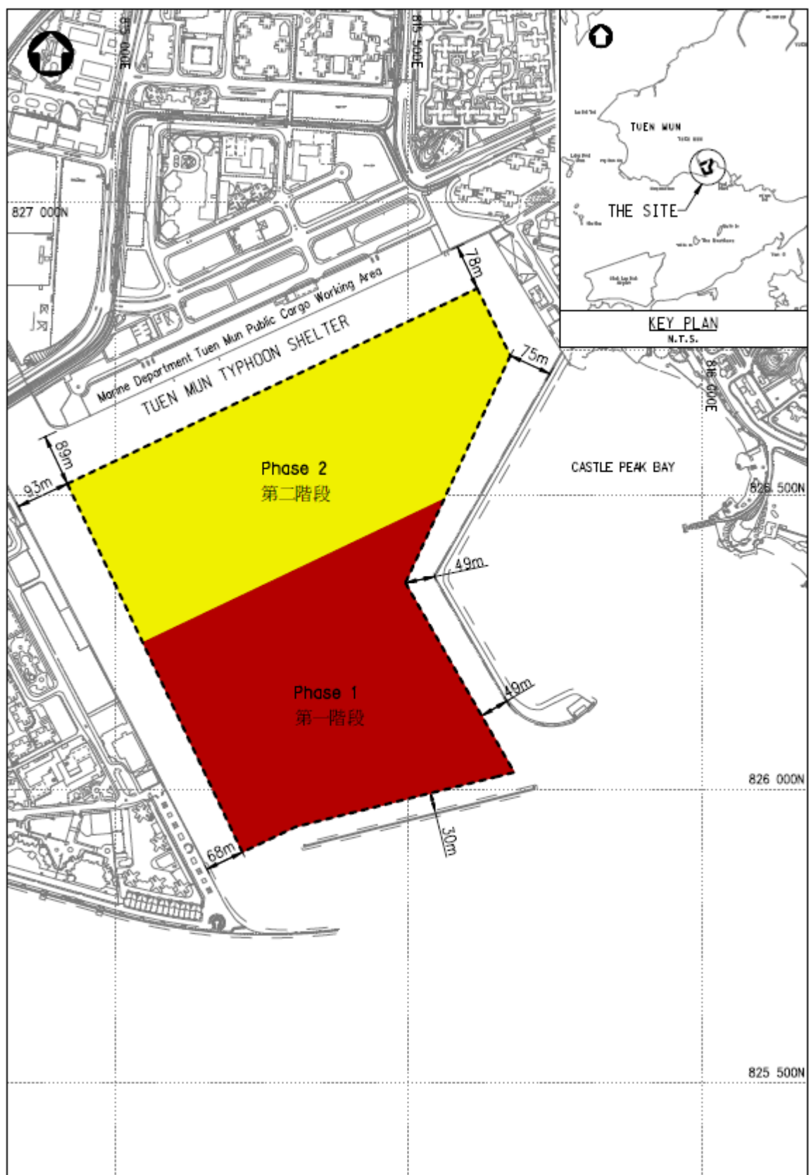
附圖一：屯門避風塘疏浚工程位置圖
