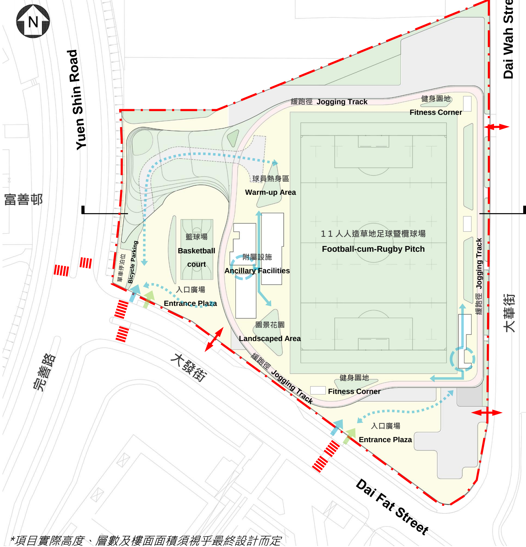
工地平面圖
