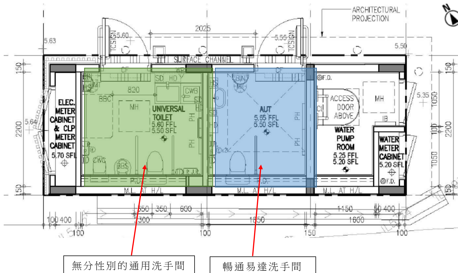
圍下村公廁翻新後的平面圖則
