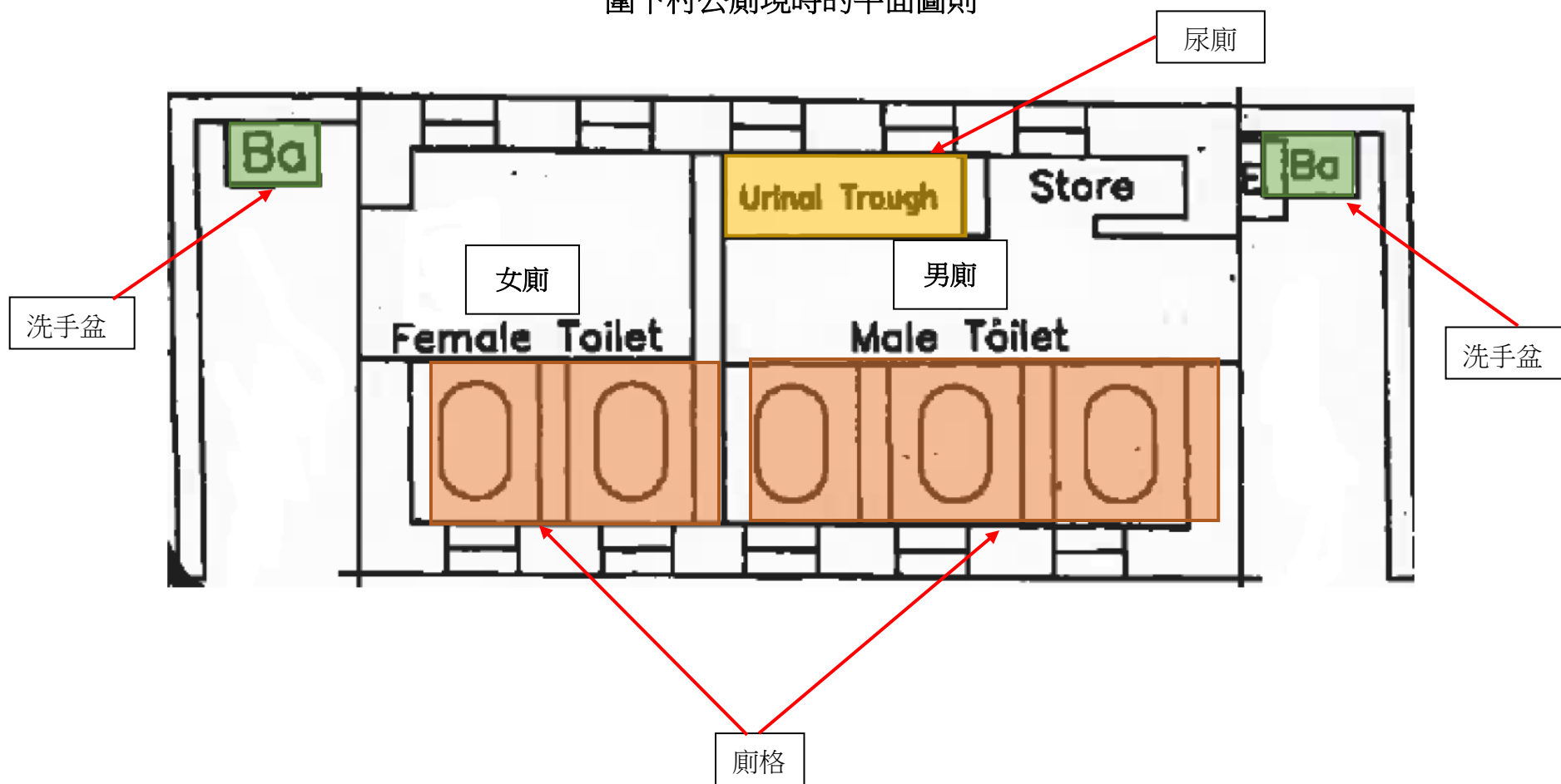
圍下村公廁現時的平面圖則
