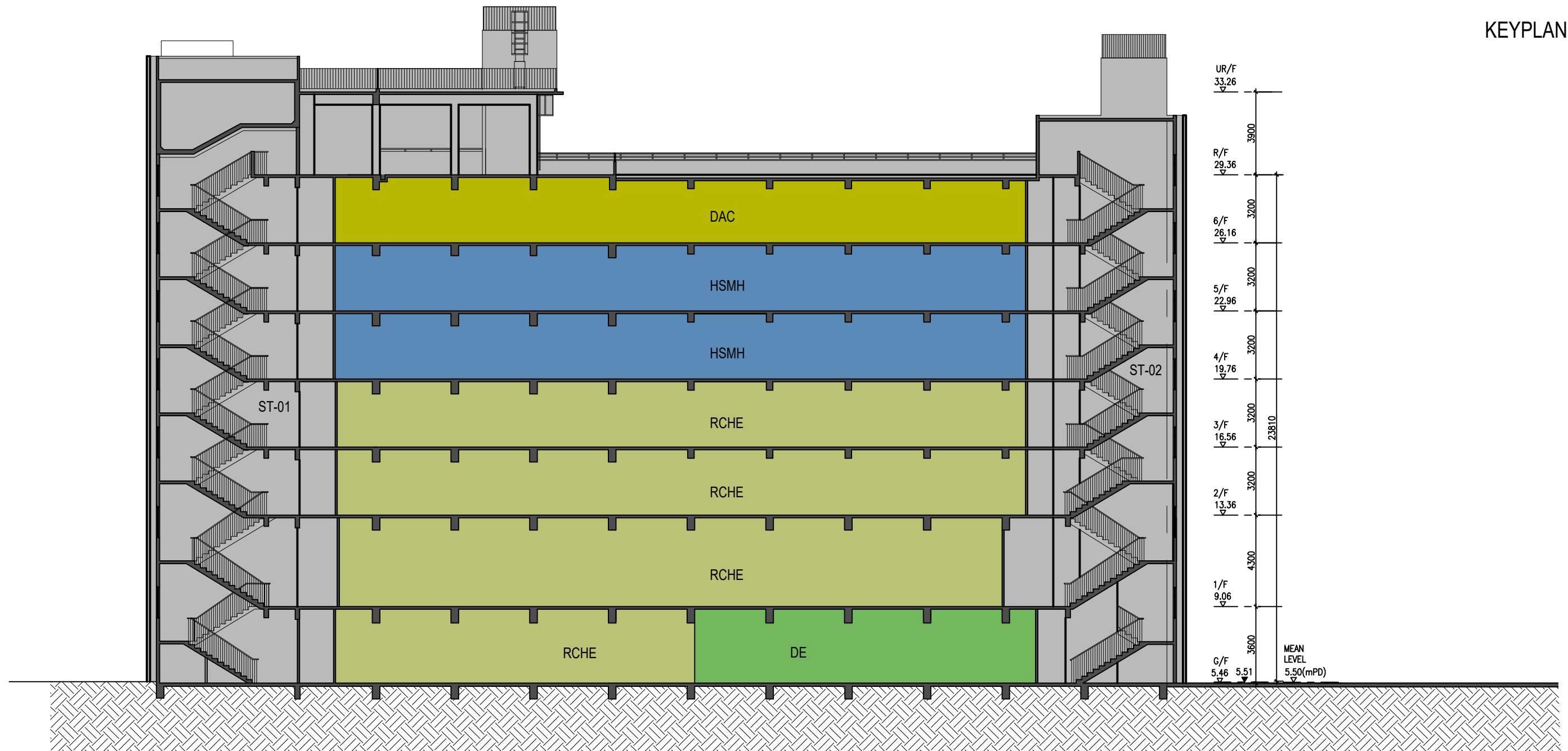
SECTION A-A
