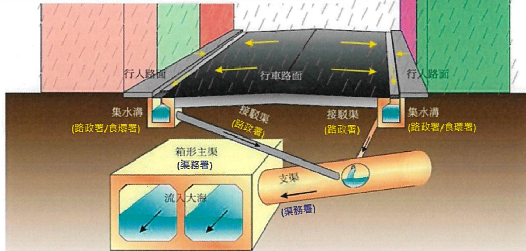
圖 1:市區雨水排放系統組合圖
