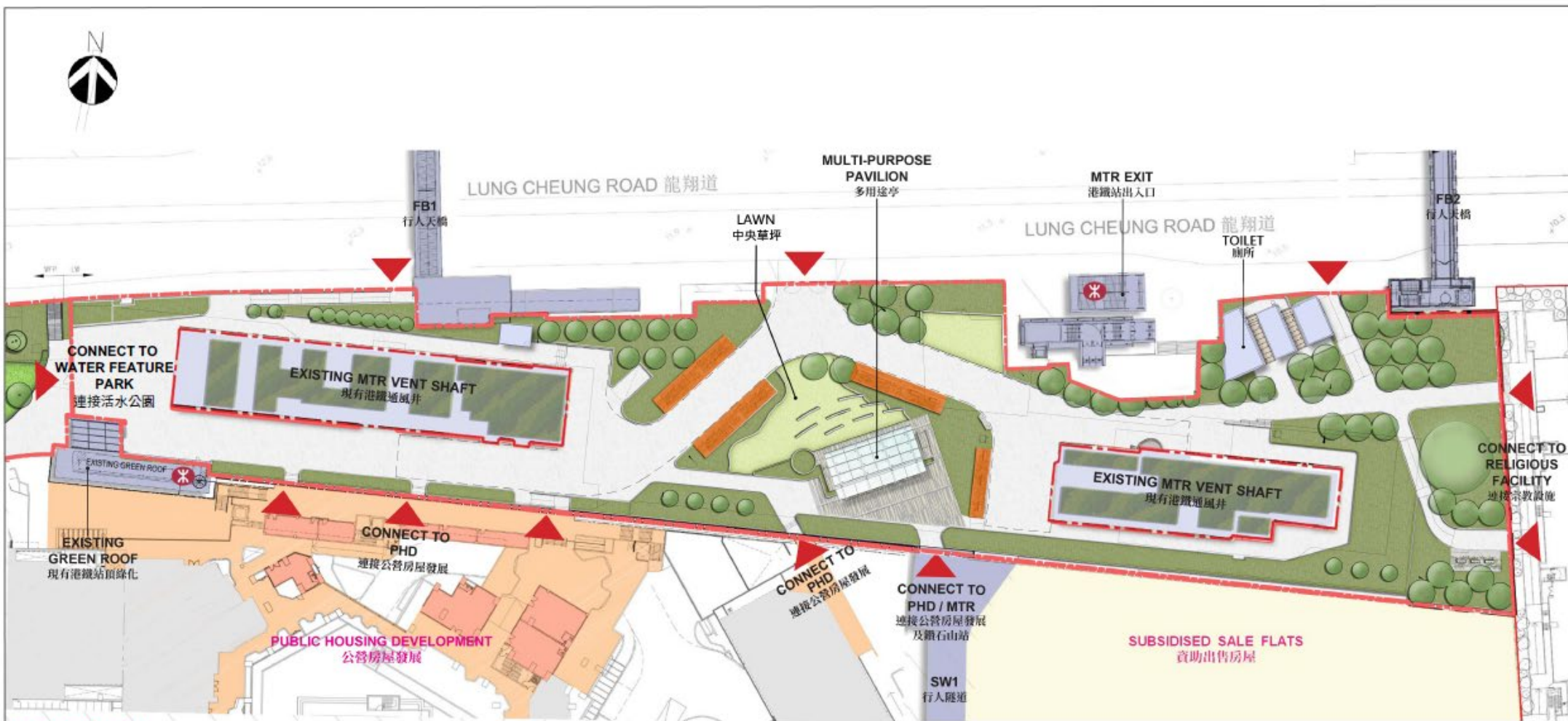
UPPER LEVEL 平台層
