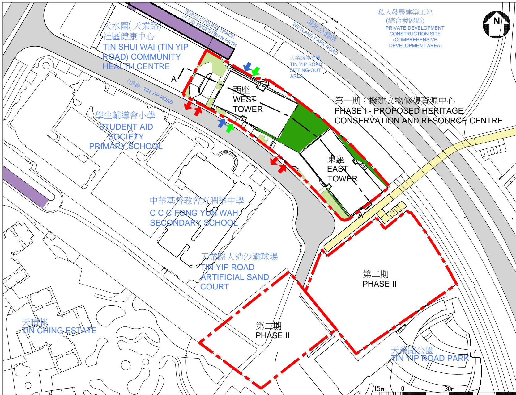
工地平面圖 SITE PLAN
