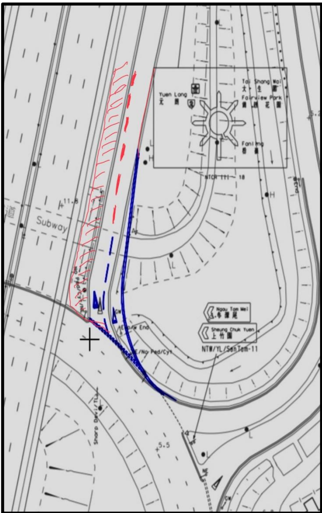
擴闊新田公路南行轉入錦綉花園迴旋處的支路
