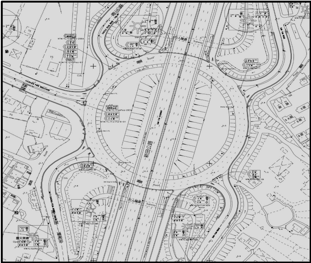
擴闊新田公路南行轉入錦綉花園迴旋處的支路
