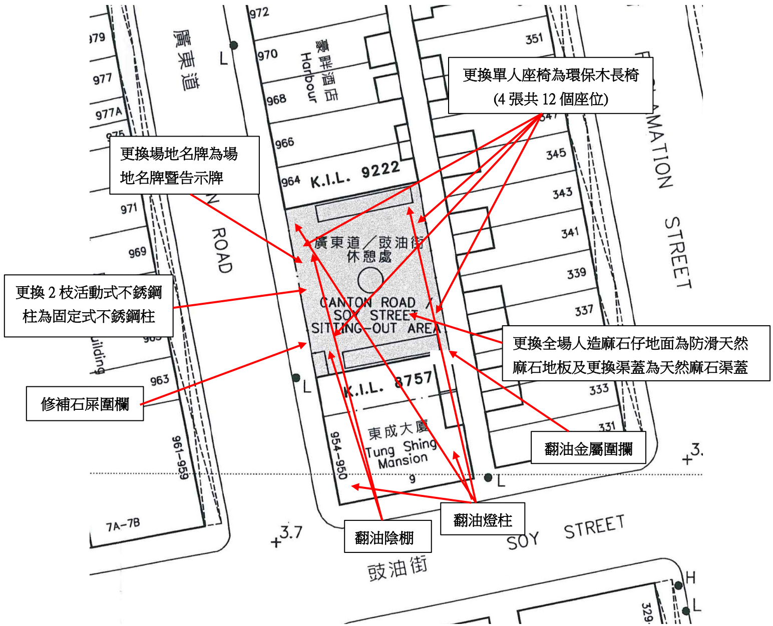
工程地點位置圖 – (b) 廣東道/豉油街休憩處
