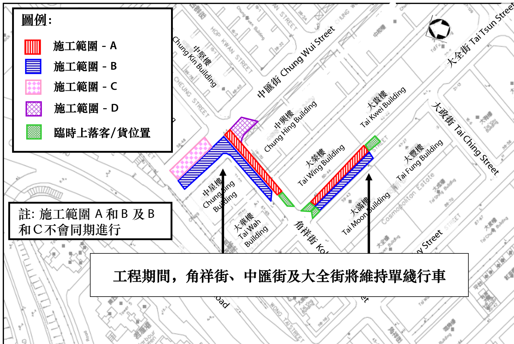
圖四 角祥街、中匯街及大全街工程之臨時交通安排
