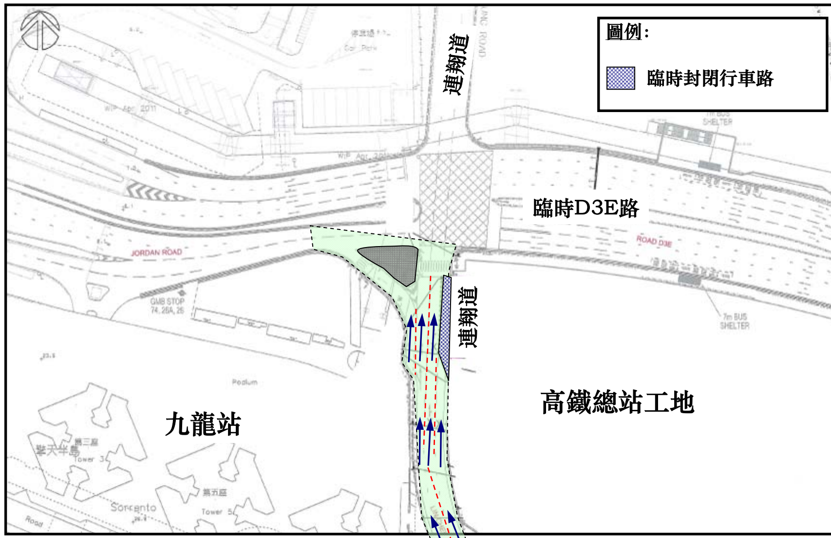
圖二 連翔道臨時交通安排
