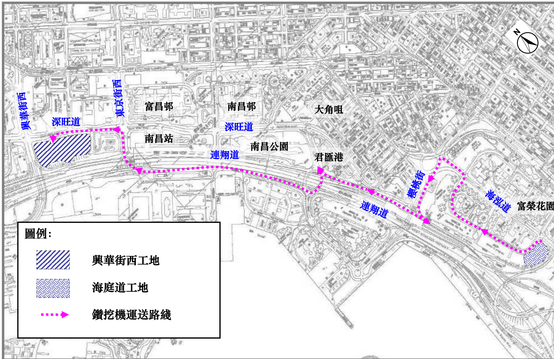
圖三 隧道鑽挖機運送路綫
